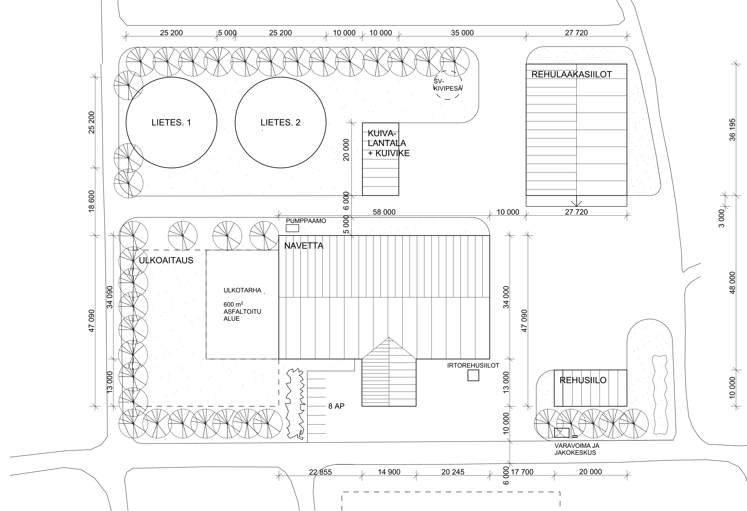
ASEMAPIIRUSTUS 1:500
